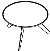
Woody Hill 02 Couchtisch Woody Hill 02 coffee table Platte mit Rahmen / plate with frame diam / diam: 55 cm Höhe / height: 37 cm / 42 cm
